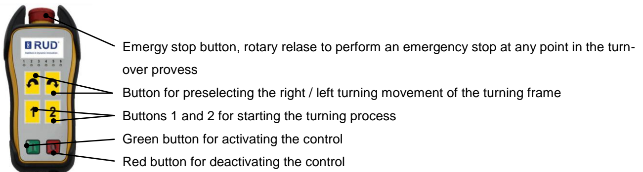
Bild 8, Remote Control
