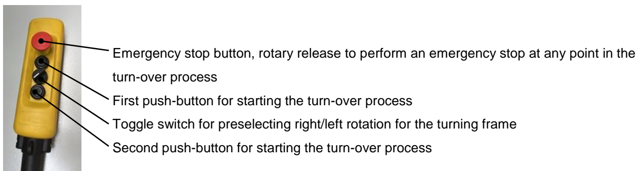
Bild 7, Control
